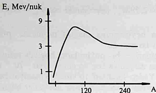
1-rasm. Solishtirma bog'lanish energiyasi ( \epsilon )ning atom massasi ( A )ga bog'liqlik grafigi
