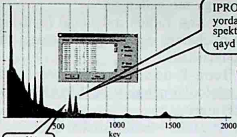
Stsintillyatsion detektor
